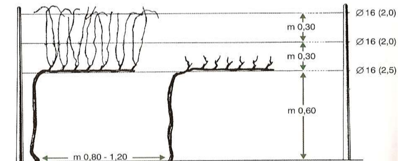
Kordon z rezniki (speronato) – pred in po zimski rezi- 14 očes
