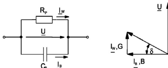
Slika: NF nadomestna shema kondenzatorja in pripadajoči kazalčni diagram
