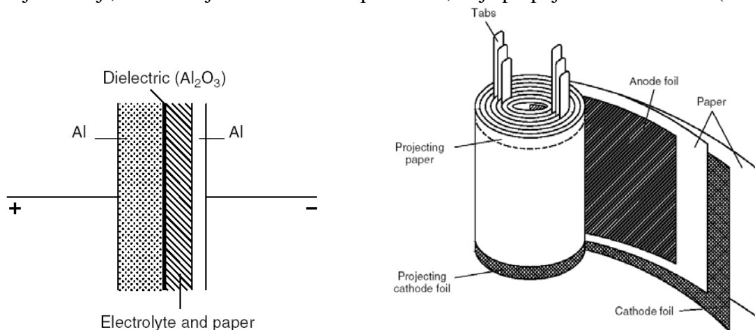
Slika: Prečni prerez in izvedba Al elektrolitskega kondenzatorja
