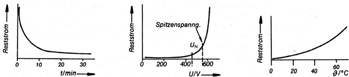
Slika: Časovna, napetostna in temperaturna odvisnost prečnega toka
