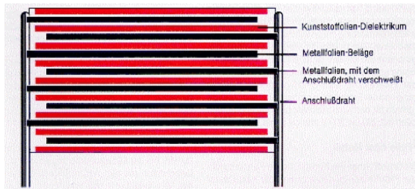
Slika: Prečni prerez nemetaliziranega folijskega kondenzatorja
