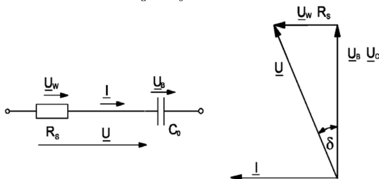
Slika: VF nadomestna shema kondenzatorja in pripadajoči kazalčni diagram
