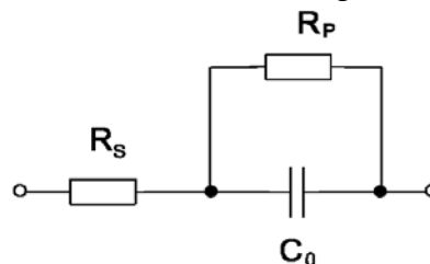
Slika: Nadomestna shema kondenzatorja z upoštevanjem upornosti priključnih vezic in končne prevodnosti dielektrika
