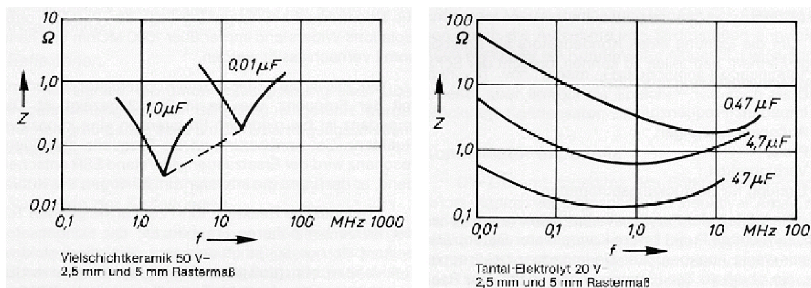
Slika: Frekvenčni potek impedanca večslojnega keramičnega in Ta-elektrolitskega kondenzatorja za različne nazivne kapacitivnosti
