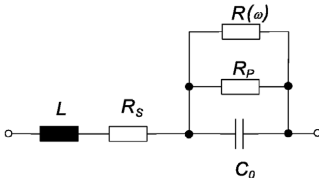
Slika: popolna nadomestna shema kondenzatorja
