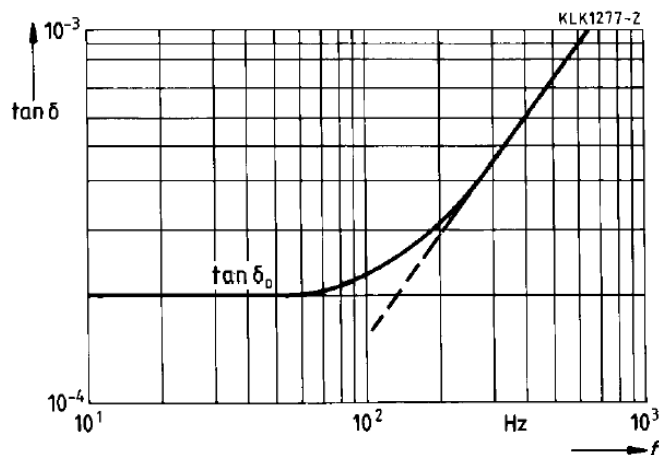
Slika: Izgubni faktor realnega kondenzatorja
