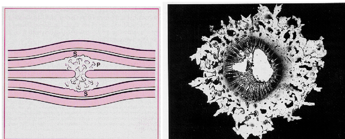
Slika: Nastanek prebojnega kanala in fotografija kanala pri realnem kondenzatorju
