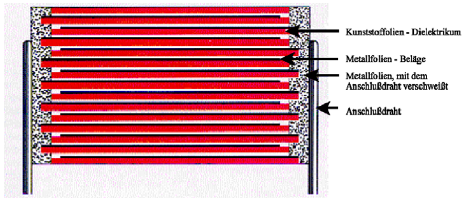
Slika: Prečni prerez metaliziranega folijskega kondenzatorja
