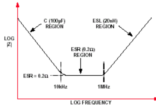
Slika: frekvenčna odvisnost Z
