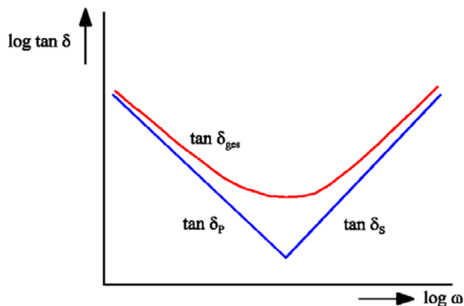
Slika: Potek izgubnega kota v odvisnosti od frekvence za idealizirani kondenzator \text{tg}\delta_{\text{GES}} (strmini premic nista prikazani v merilu)
