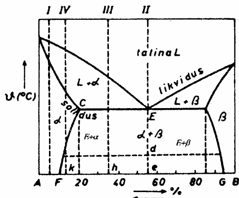
Slika 4.7 Fazni diagram pri delni topnosti
