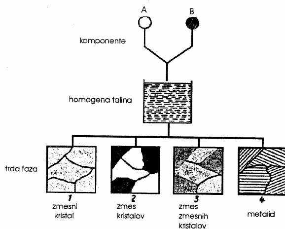
Slika 4.2 Produkti homogene taline
