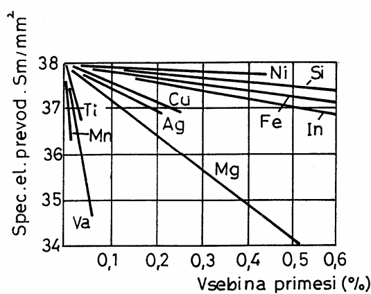
Slika 4.14 Vpliv primesi na specifično prevodnost aluminija
