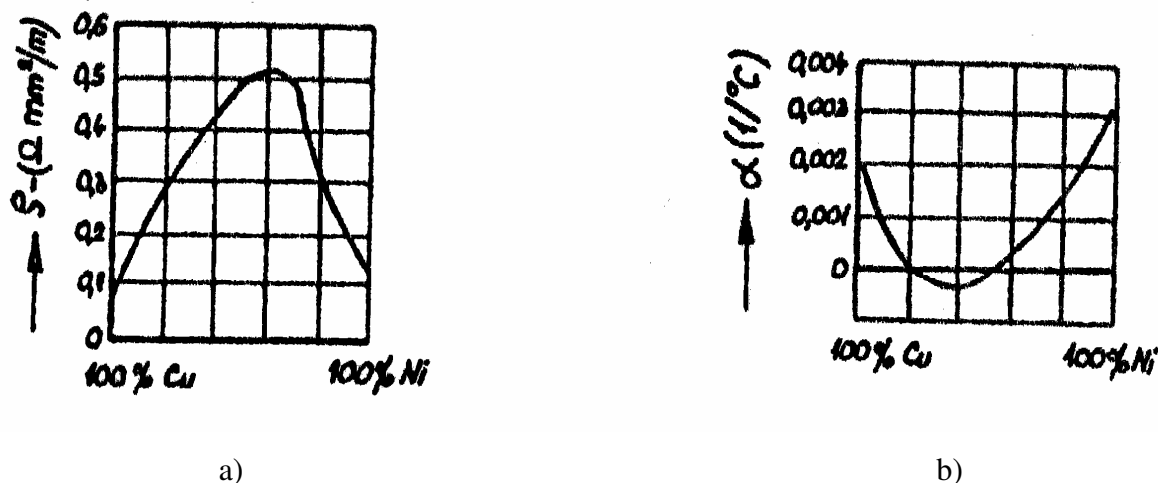
Slika 4.8 Potek upornosti pri različnih koncentracijah komponent v zlitini a), potek temperaturnega koeficienta upornosti v odvisnosti od koncentracije komponent v zlitini b)
