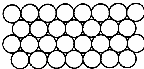
Slika 3.10 Razporeditev gradnikov
