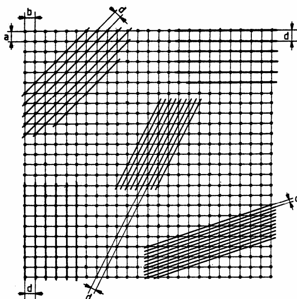
Slika 3.2 Mrežne ravnine
