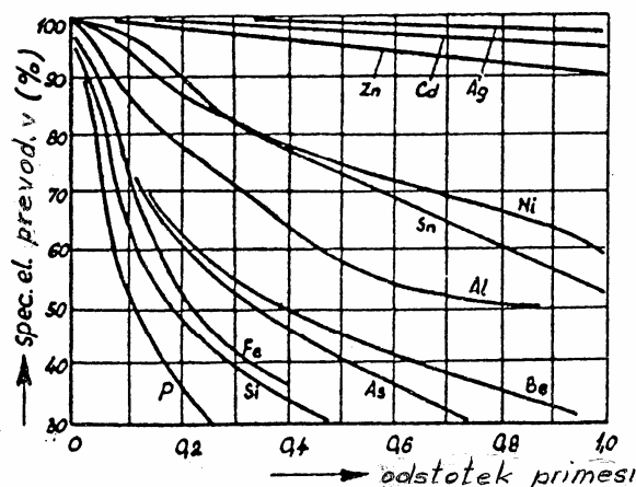
Slika 4.10 Vpliv primesi na specifično prevodnost bakra
