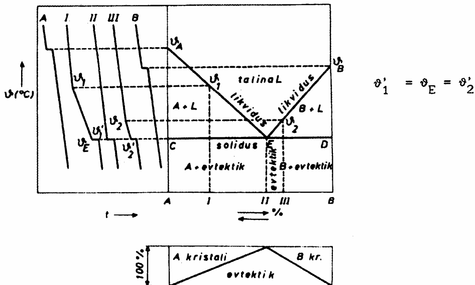
Slika 4.5 Fazni diagram sistema pri popolni netopnosti
