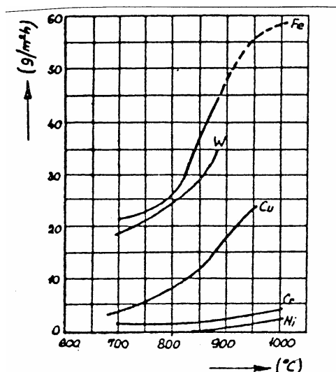
Slika 4.9 Oksidacija kovin v odvisnosti od temperature
