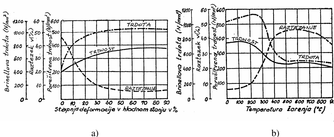
Slika 4.11 Vpliv hladne obdelave na mehanske lastnosti bakra a) in vpliv toplotne obdelave b)
