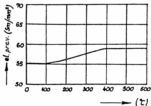
Slika 4.12 Vpliv toplotne obdelave bakra na specifično električno prevodnost
