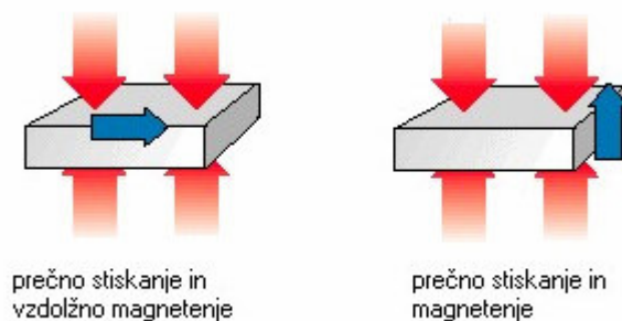
Slika 5.69 Oblikovanje magnetnih jeder v magnetnem polju.
