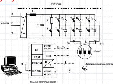
Slika 13. 1: Karakteristična konfiguracija modernega pogona z asinhronskim motorjem
