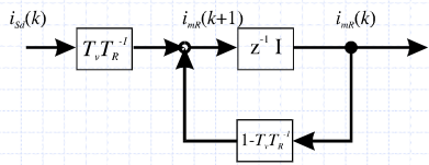
Slika 12. 4: Diskretni model generiranja fluksa v KSP
