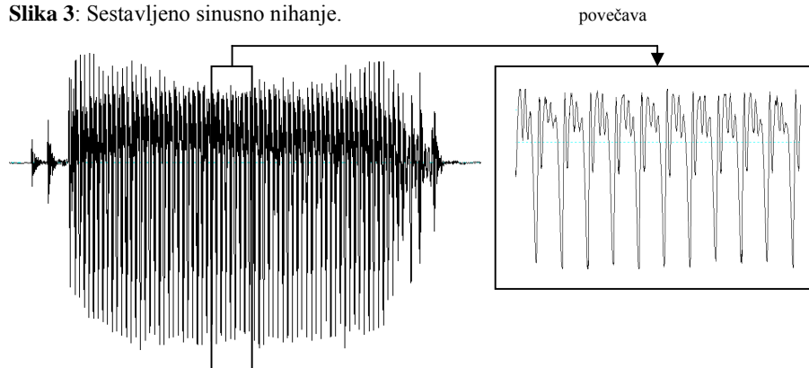
Slika 3: Sestavljeno sinusno nihanje.
