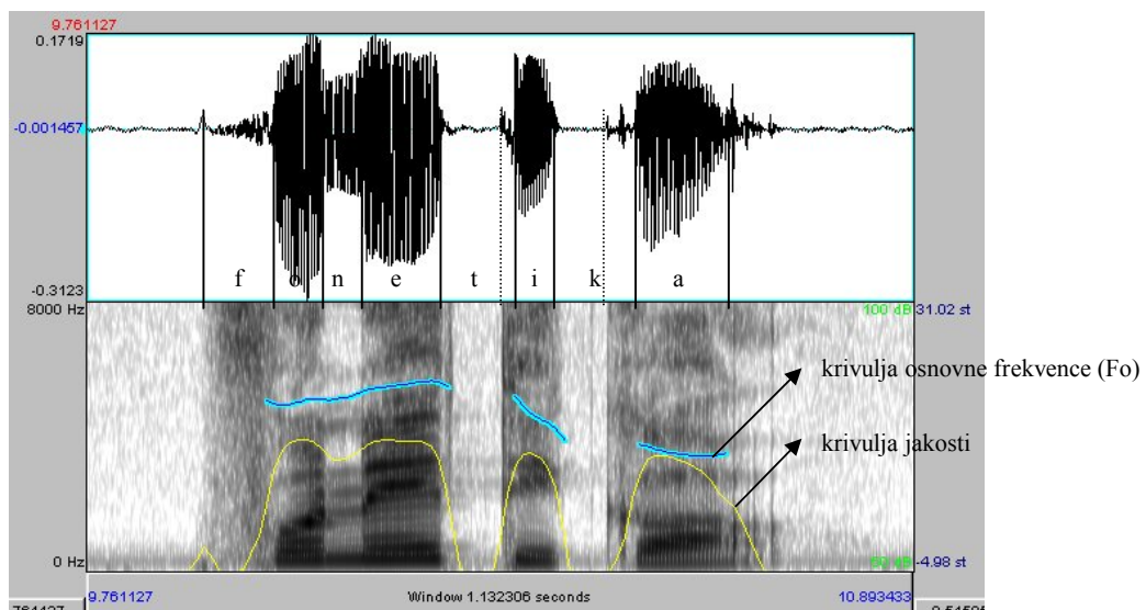
Spektrogram 3: Segmentiranje in računalniško podana osnovna frekvenca ter jakost glasov.
