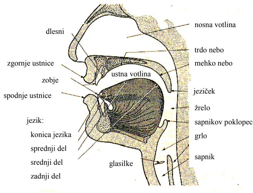
Slika 2: Struktura govornega trakta od ustne in nosne votline do grla z glasilkami.
