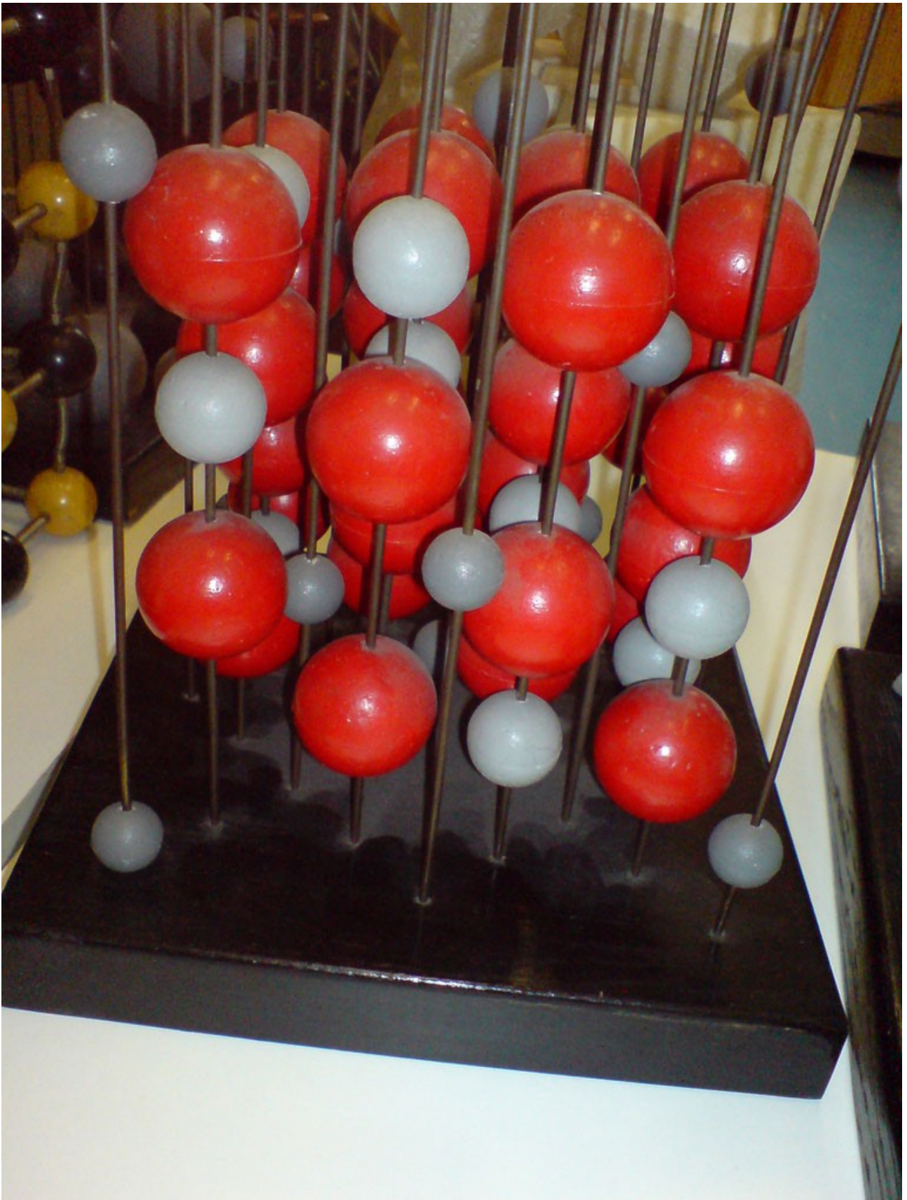
MgAl 2 O 4 - spinel
