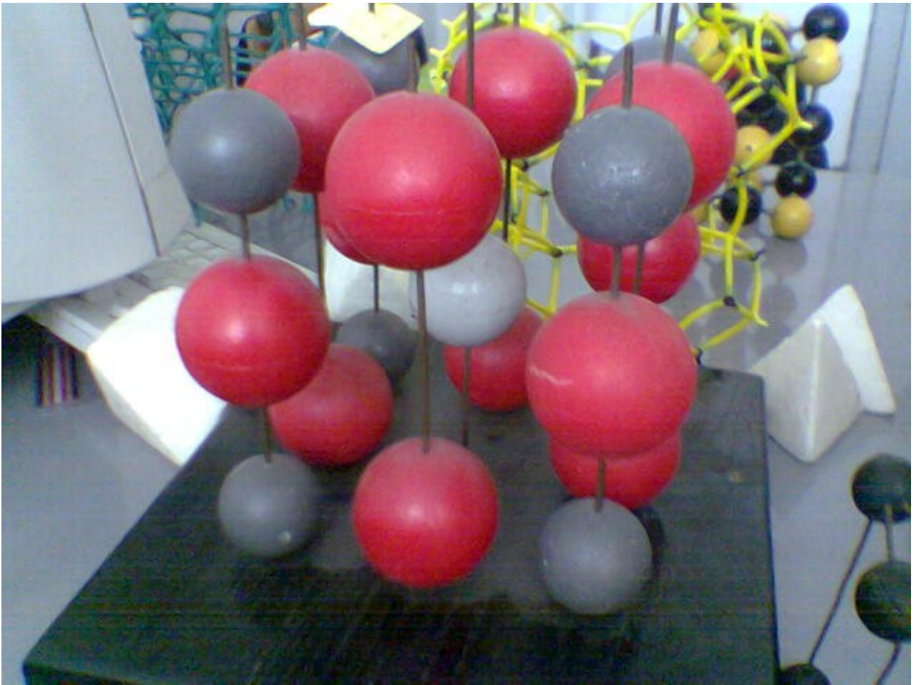
CaTiO 3 - perovskit
