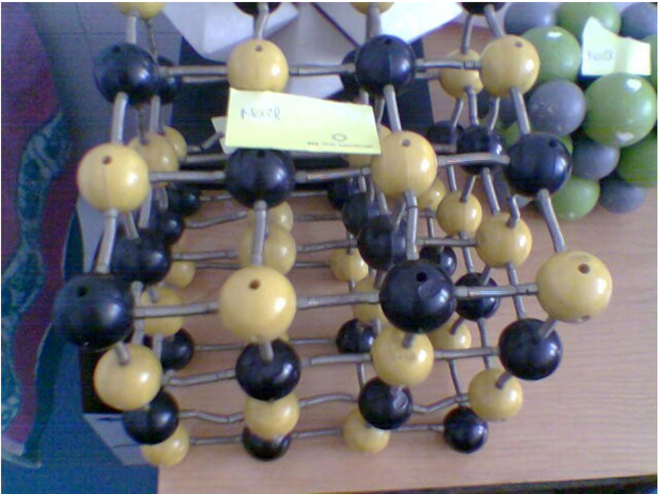
NaCl
