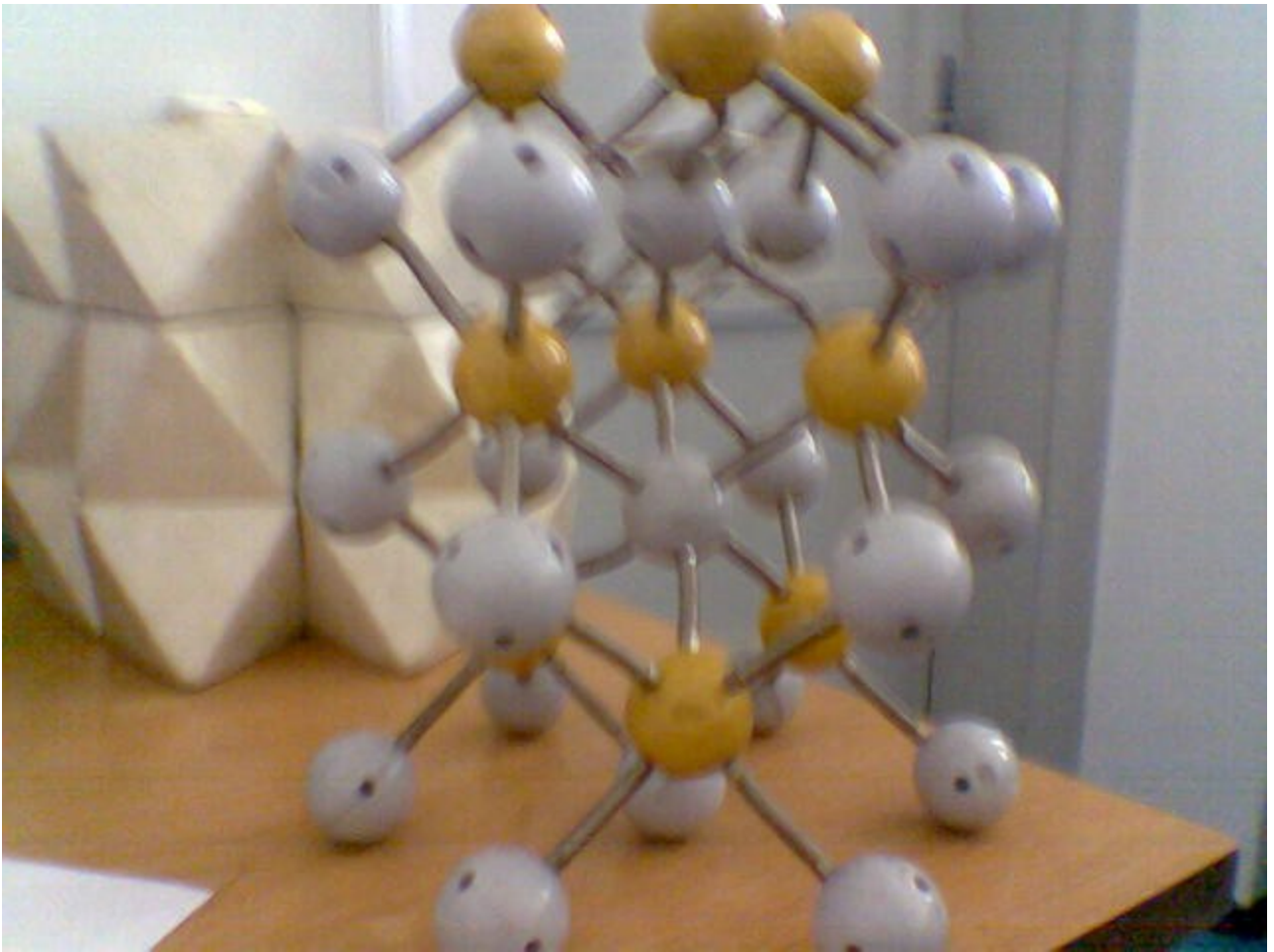
NiAs
