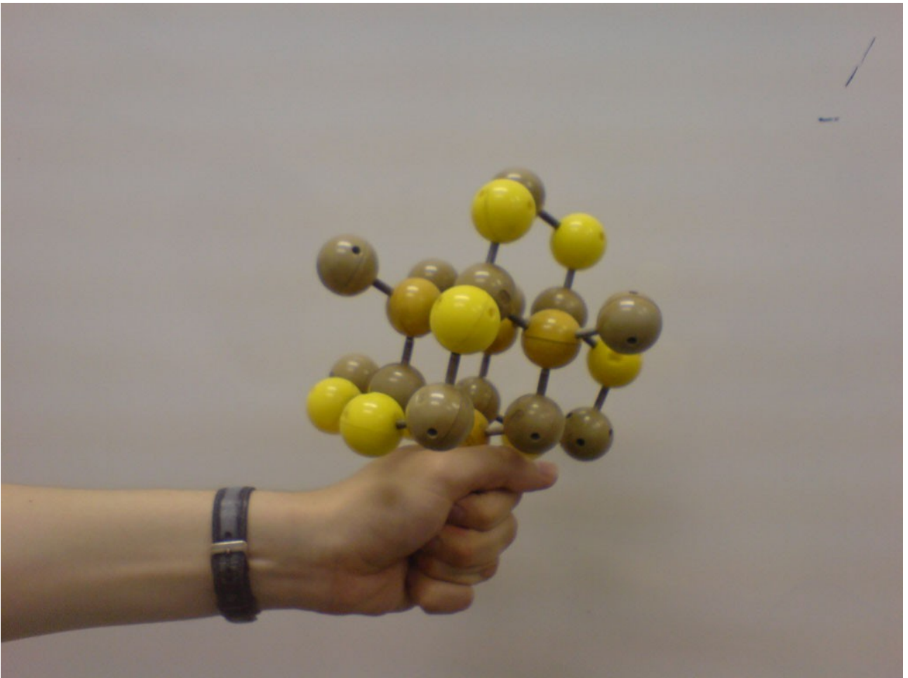
ZnS - sfalerit
