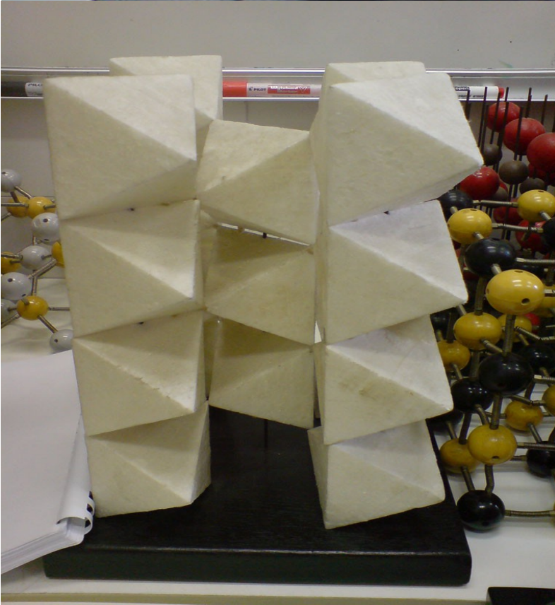
TiO 2 - rutil
