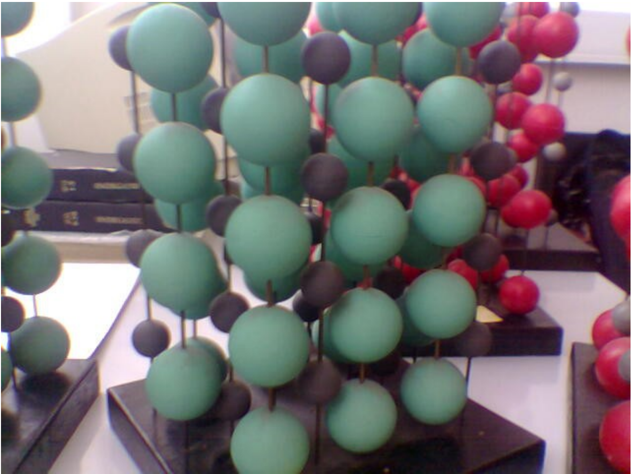
\text{CuCl}_2
