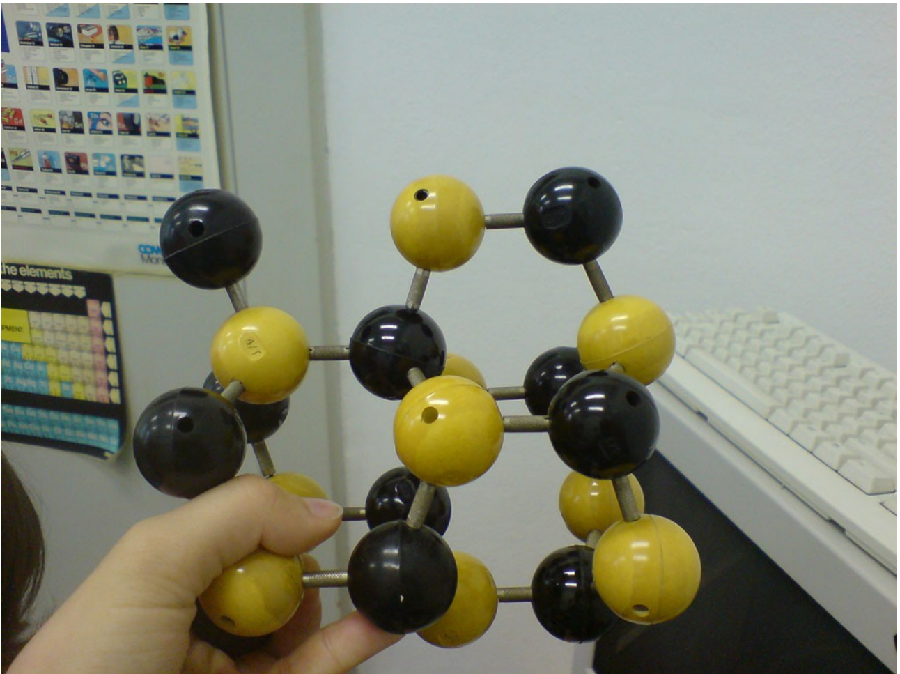
ZnS - wurzit
