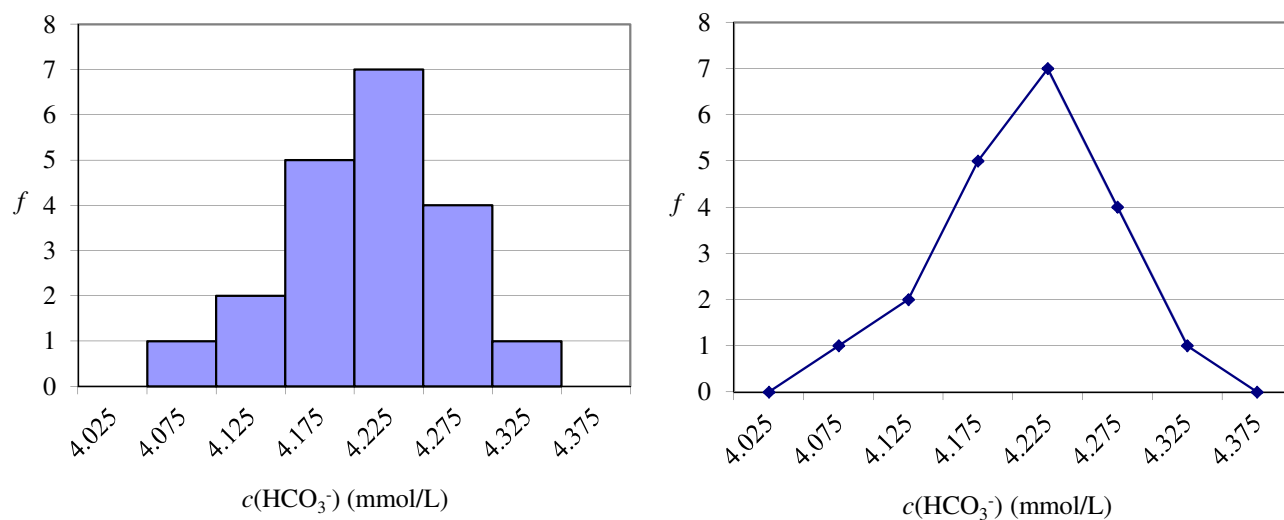
Slika 1. Grafični prikaz frekvenčne porazdelitve rezultatov (levo frekvenčni histogram, desno frekvenčni poligon)
