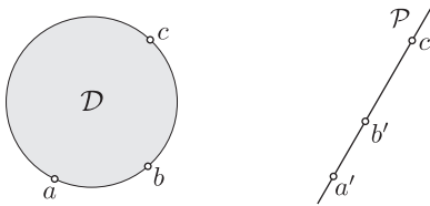
Slika 6.19: Transformacija \varphi preslika krog na premico
