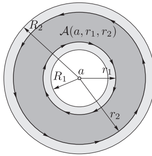
Slika 6.13: Kolobar \mathcal{A}(a, r_1, r_2)
