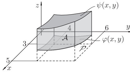
Slika 3.12: Skica za zgled 3
