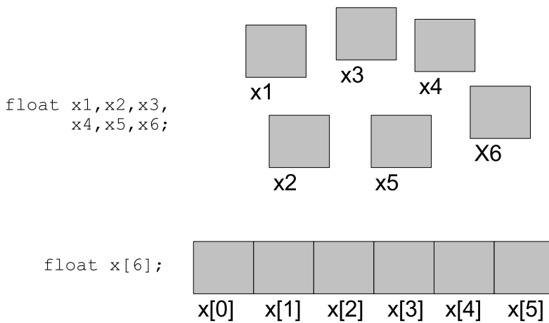
Slika 5.1: Deklaracija spremenljivk - brez in z uporabo tabele (shematski prikaz)
