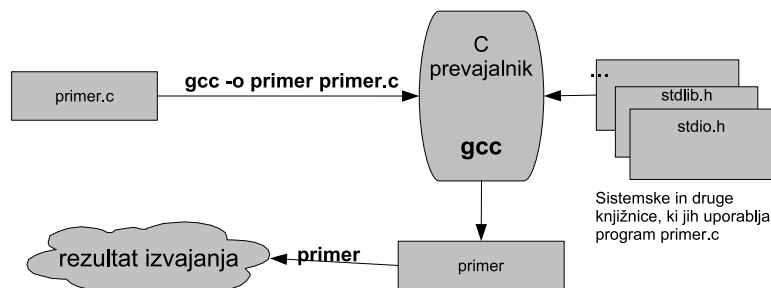
Slika 1.2: Primer prevajanja in izvajanja v C
