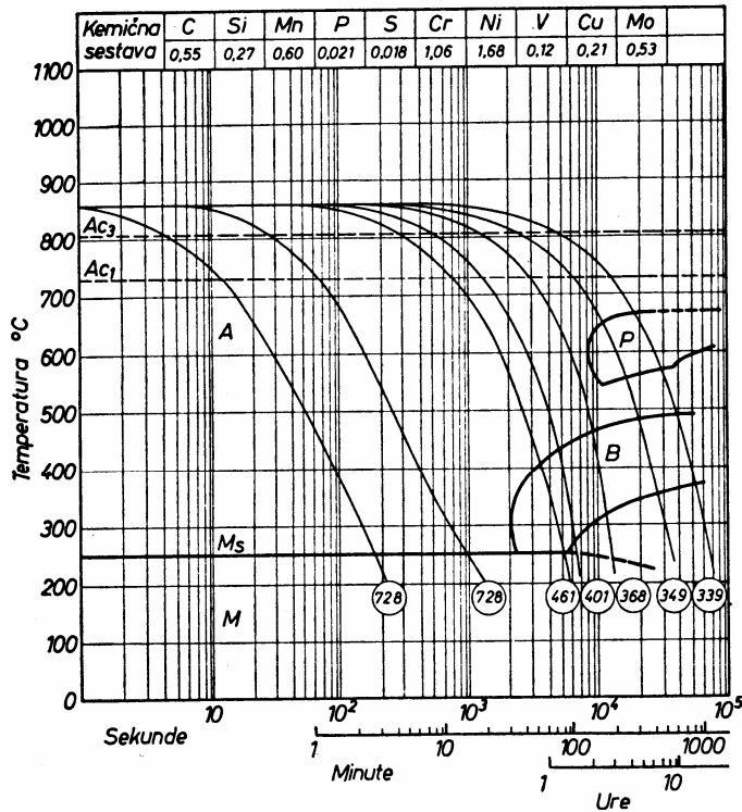
Slika 7. Krivulje TTT za jekli C 45 (Č 1530) in UTOP ekstra 2
