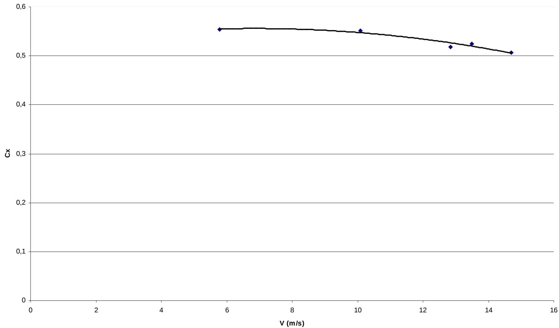
Diagram spremembe koeficienta upora v odvisnosti od hitrosti toka:
