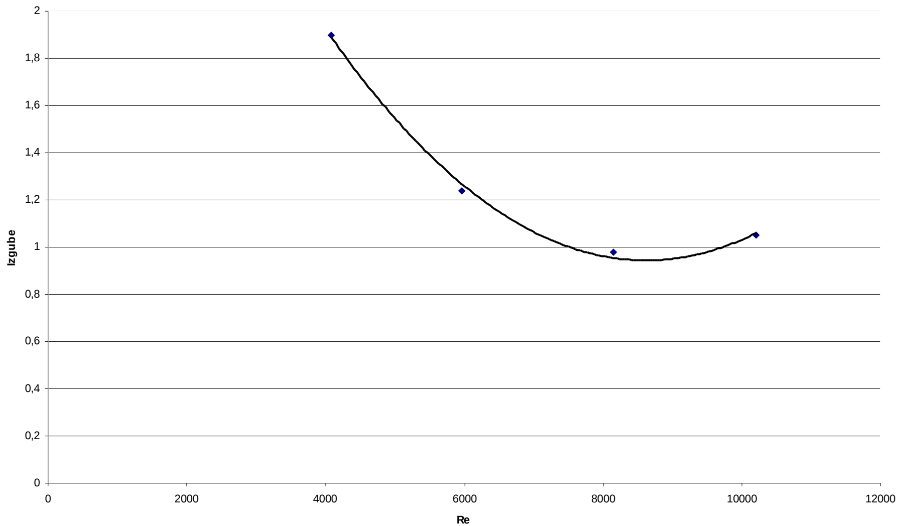
Diagram spremembe lokalnih izgub enega kolena v odvisnosti od Reynoldsovega števila:
