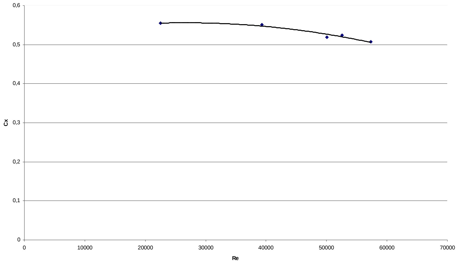
Diagram spremembe koeficienta upora v odvisnosti od Reynoldsovega števila:
