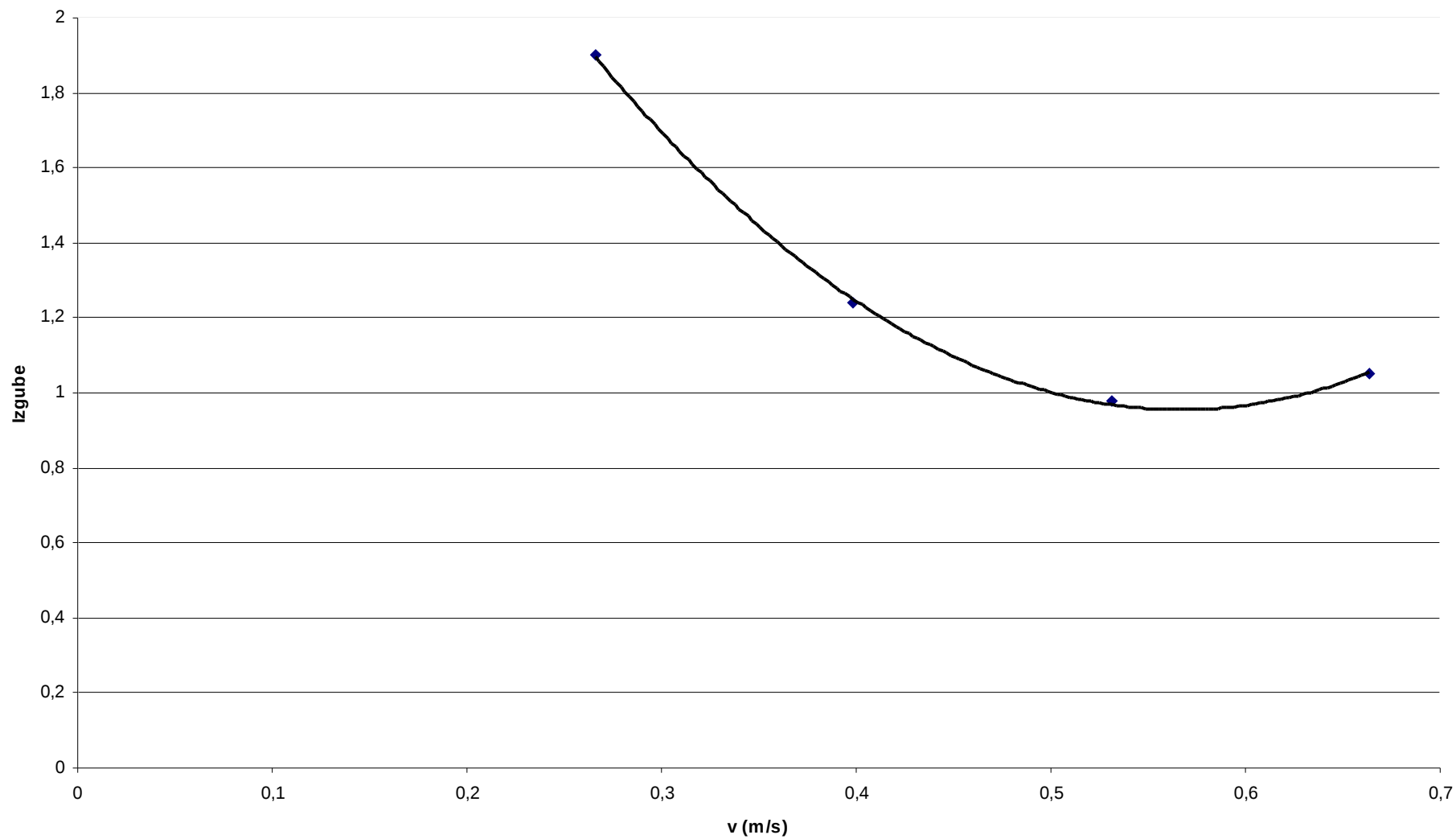
Diagram spremembe lokalnih izgub enega kolena v odvisnosti od hitrosti toka:
