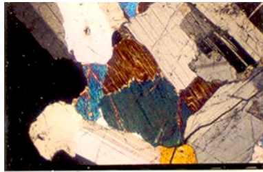
Slika 9 Anhedralna zrna monoklinskega piroksena
