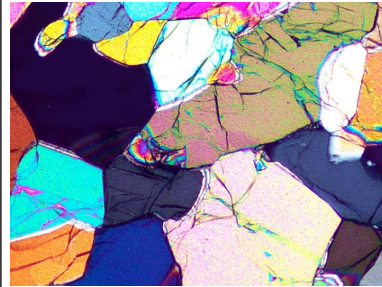
Slika 10 Enakomerno zrnata struktura
