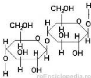
Celuloza
