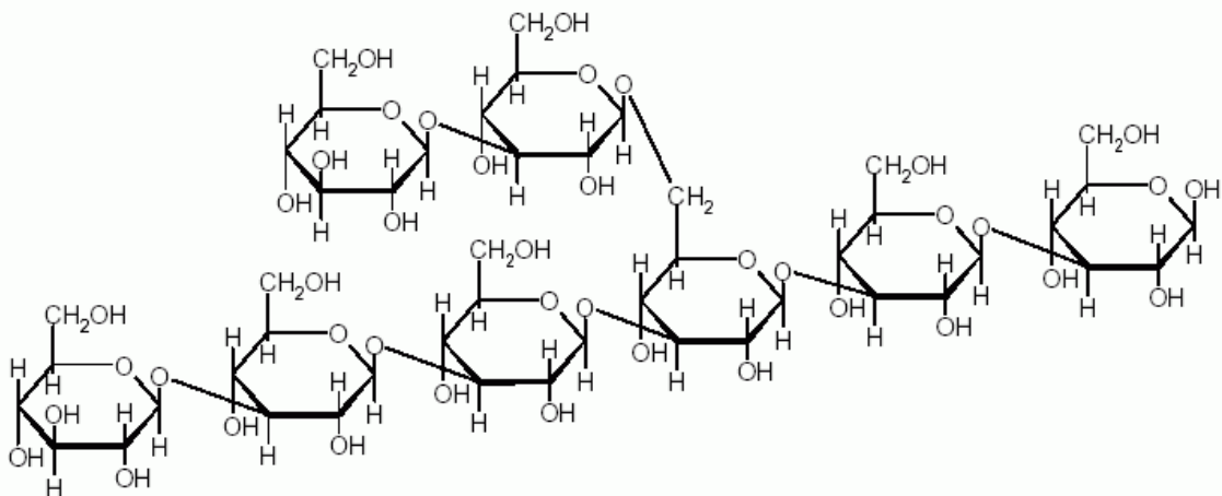
Škrob
