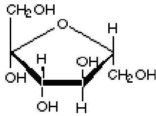
Fructose
