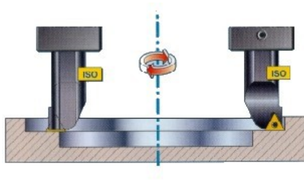
GREZILO Z VSTAVLJENIMI STRUŽNIMI NOŽI
